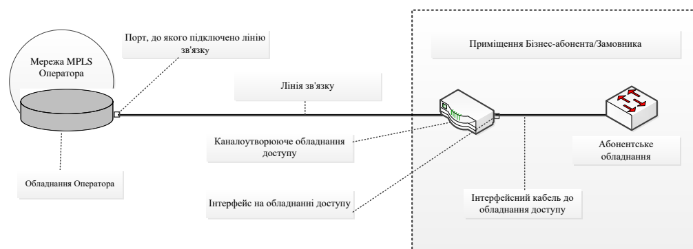
Рис. Конфігурація обладнання та відповідальність Сторін (зони відповідальності Сторін зазначаються у Заяві-присднанні)
